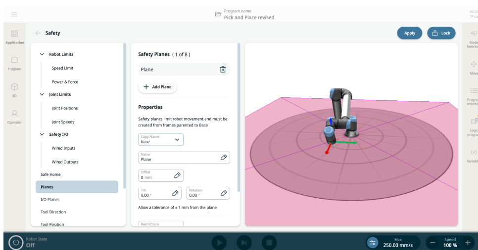
Číslo 1.5: Obrazovka PolyScope X zobrazující bezpečnostní roviny.
