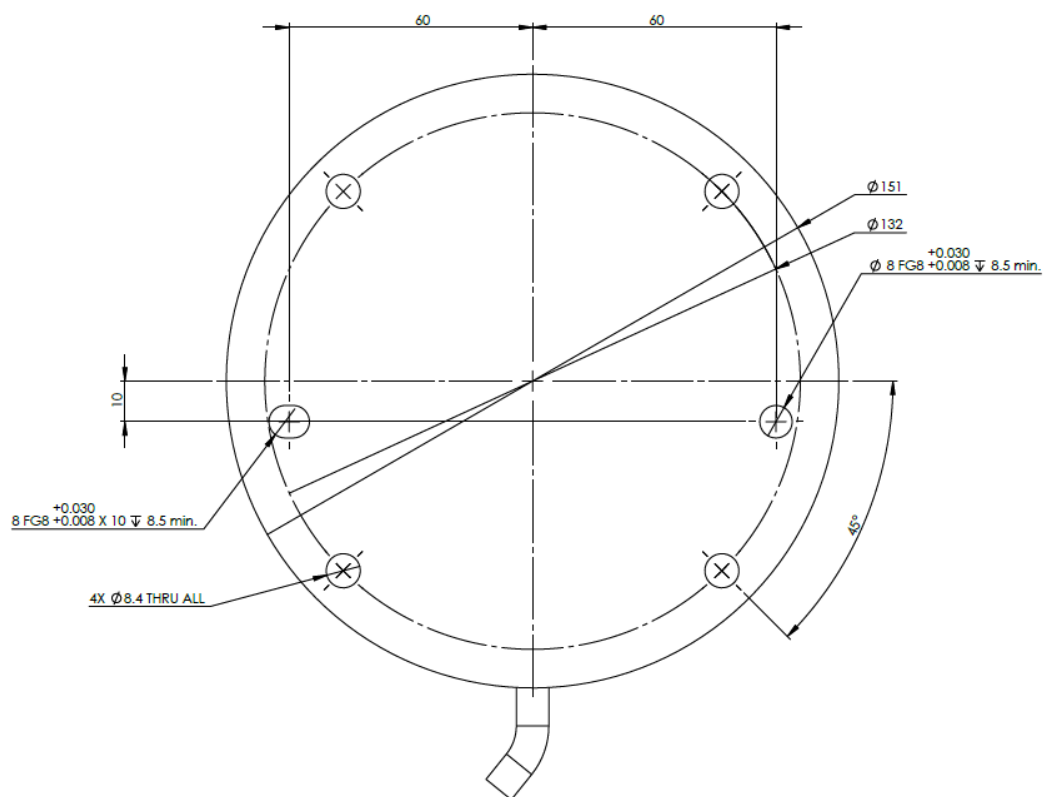
1.1: Pohled na základnu robota zespodu
